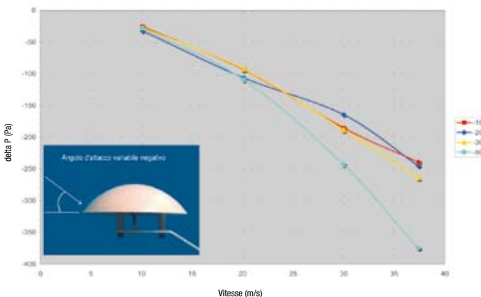
\Delta P selon la variation de l'angle d'embardeé \beta (angle de jonction \alpha = 0^\circ )
