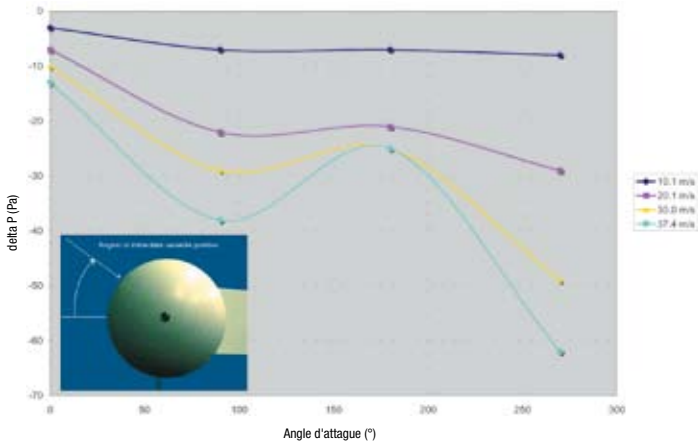
\Delta P selon la variation de l'angle de jonction \alpha (angle d'embardeé \beta = 0^\circ )
