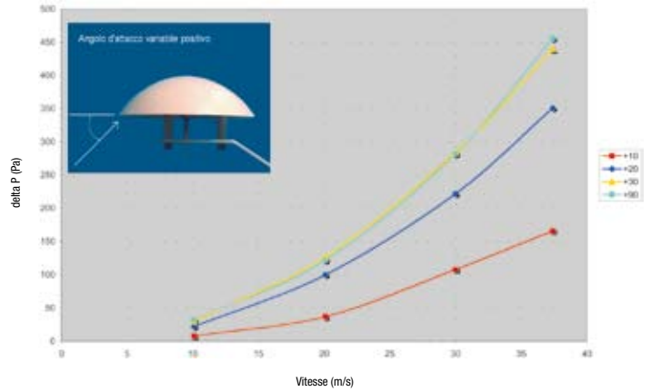
\Delta P selon la variation de l'angle d'embardeé \beta
